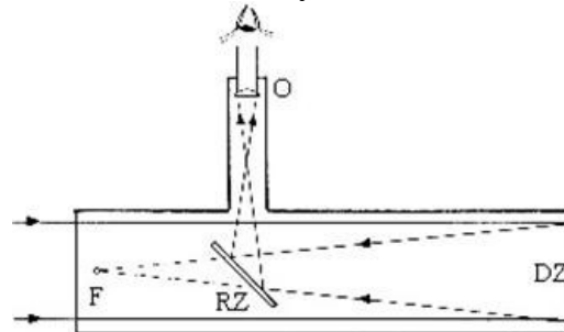
Newtonův zrcadlový dalekohled
